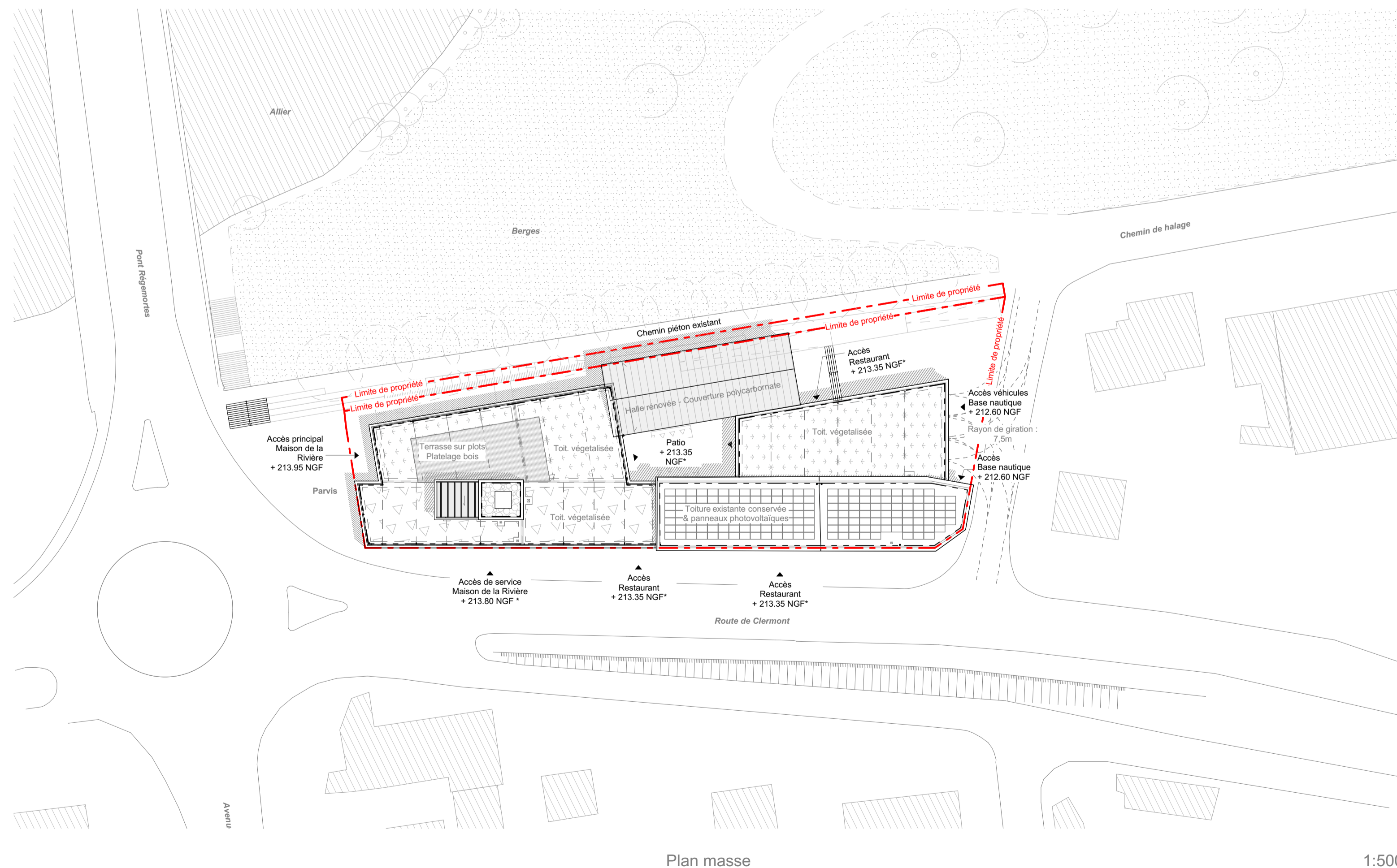
Plan masse
